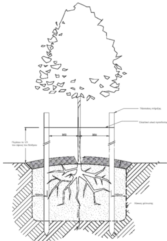
Σχήμα 3 - Στήριξη με δύο κατακόρυφους πασσάλους.
